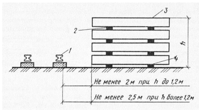
Рис. 2. Схема размещения штабелей грузов у железнодорожного или кранового пути 1 — головка рельса; 2 — прокладка; 3 — груз; 4 — подкладка
